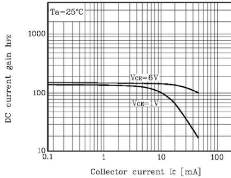
hFE - Ic
