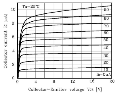
Ic - Vce
